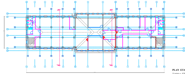
PLAN ETAJ 2 S totala = 676 MP
