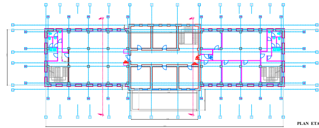
PLAN ETAJ 1 S totala = 745 MP din care S terasa = 69 MP
